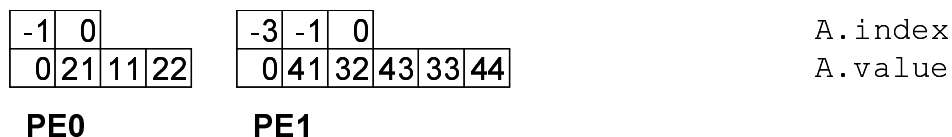
図 11: DIA 形式のデータ構造 (マルチプロセス環境)
